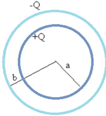
Figura 1: Figura 1: Capacitor esférico
